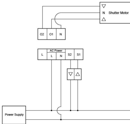
Verkabelung 1:
