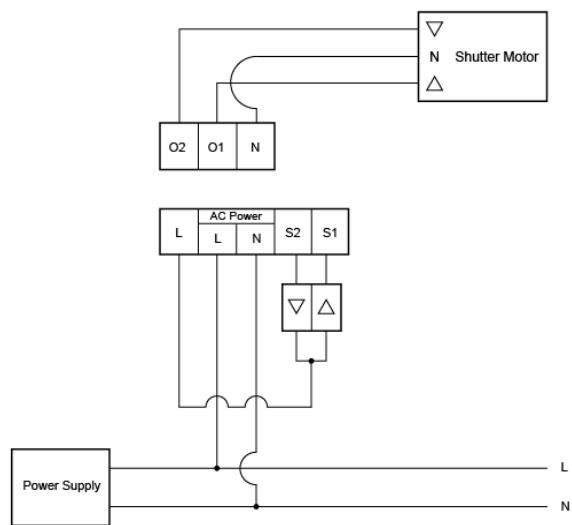
Verkabelung 2:
